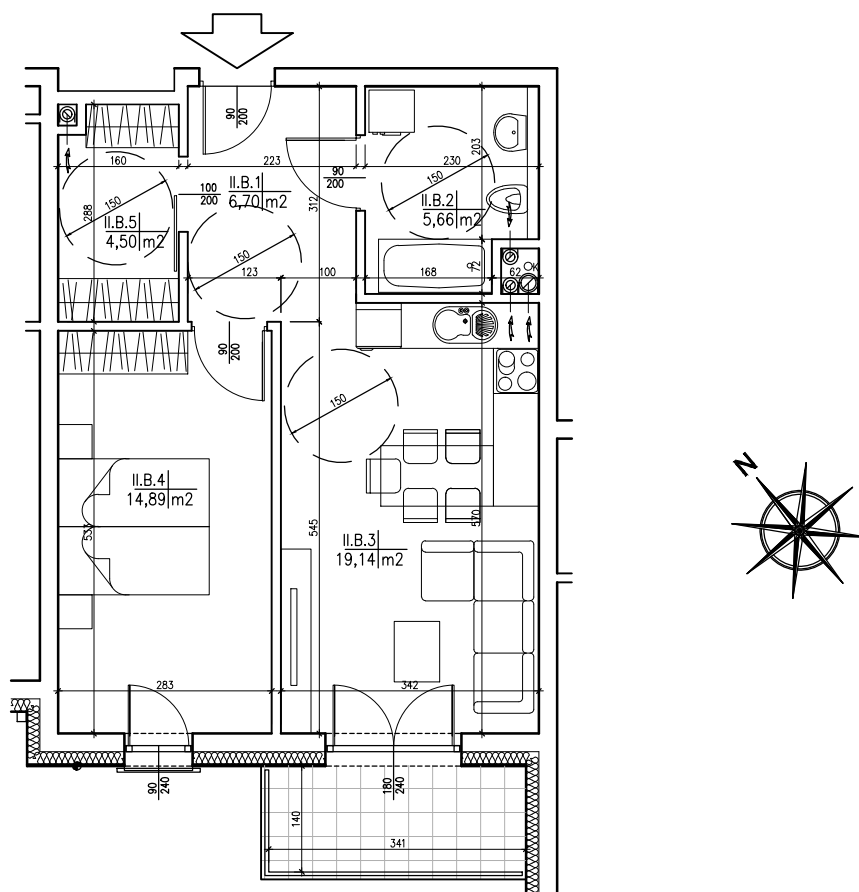
ZESTAWIENIE POMIESZCZEŃ – MIESZKANIE "2B"
